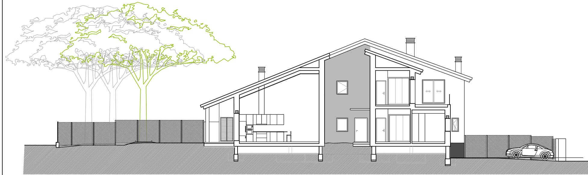
SECCIÓN ESQUEMÁTICA
