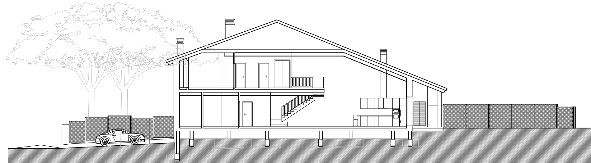
SECCIÓN ESQUEMÁTICA
