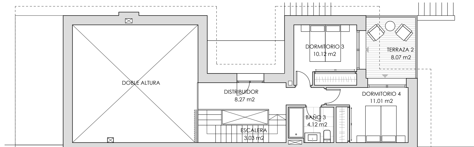
PLANTA PRIMERA
