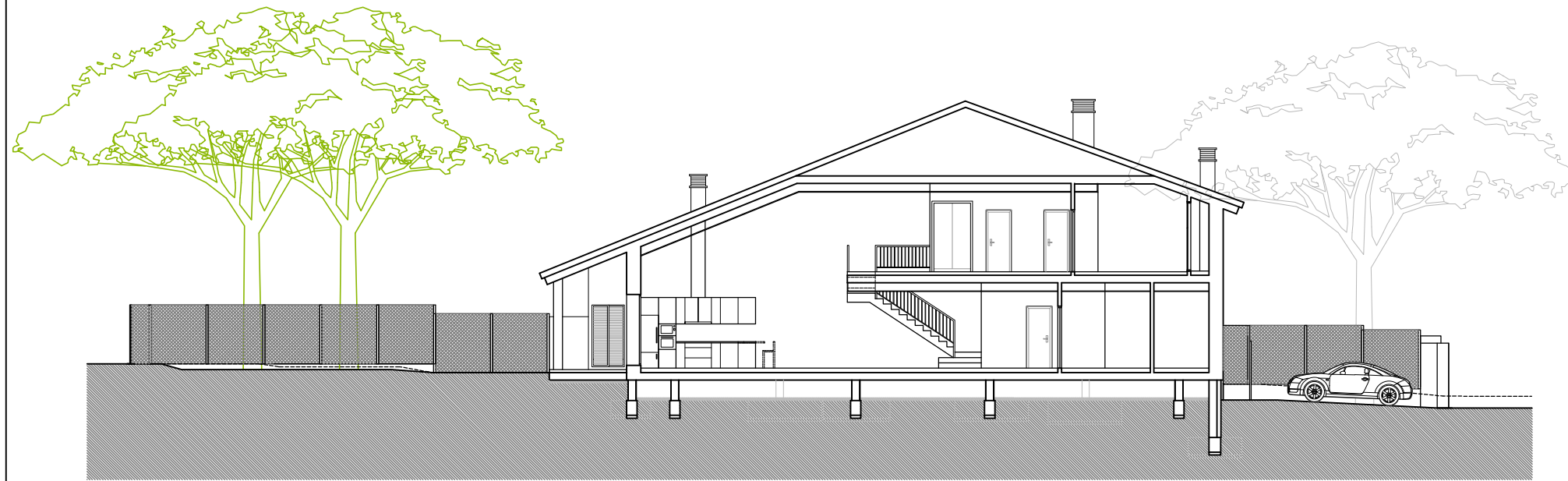
SECCIÓN ESQUEMÁTICA
