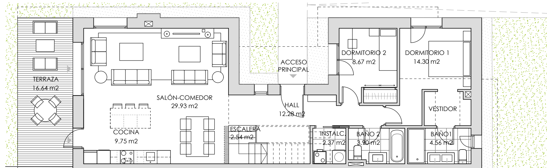
PLANTA BAJA
