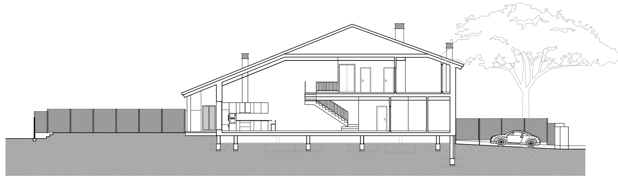
SECCIÓN ESQUEMÁTICA
