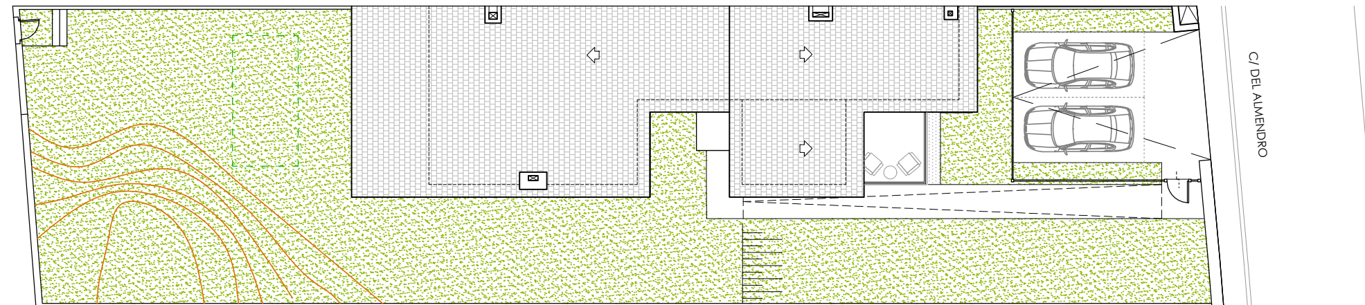
PLANTA CUBIERTA
