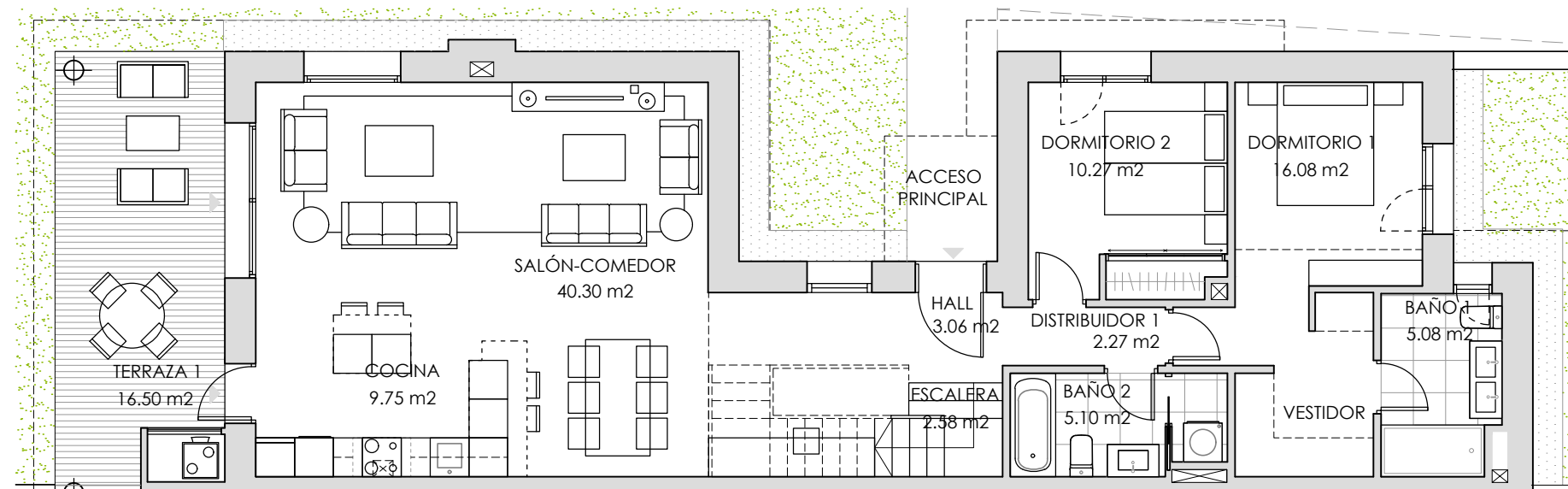
PLANTA BAJA
