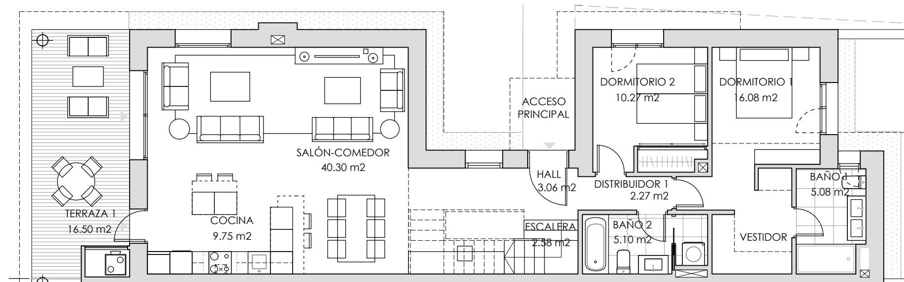
PLANTA BAJA
