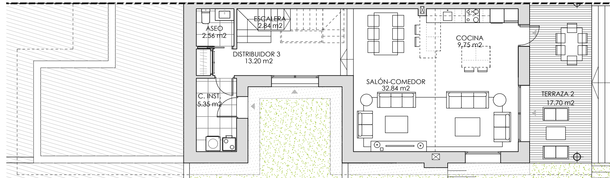
PLANTA BAJA
