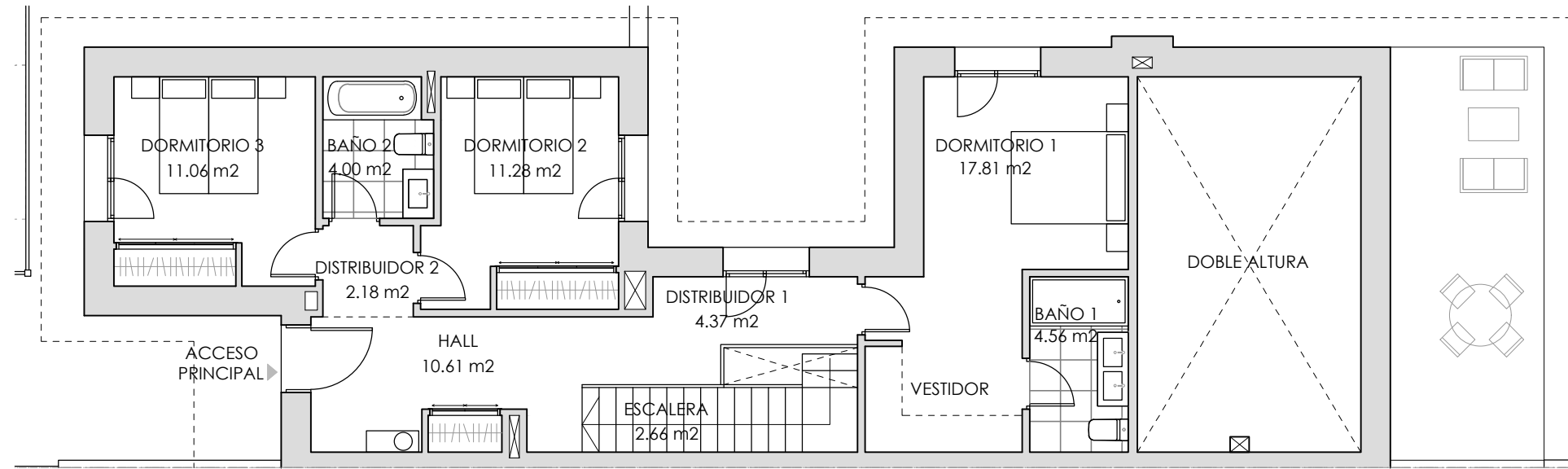
PLANTA PRIMERA
