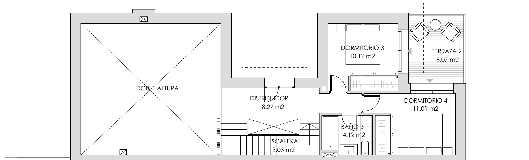
PLANTA PRIMERA
