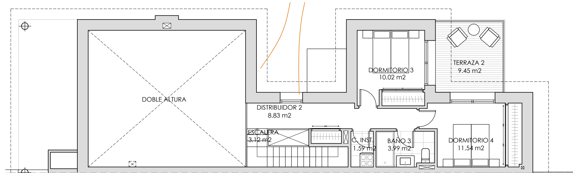
PLANTA PRIMERA
