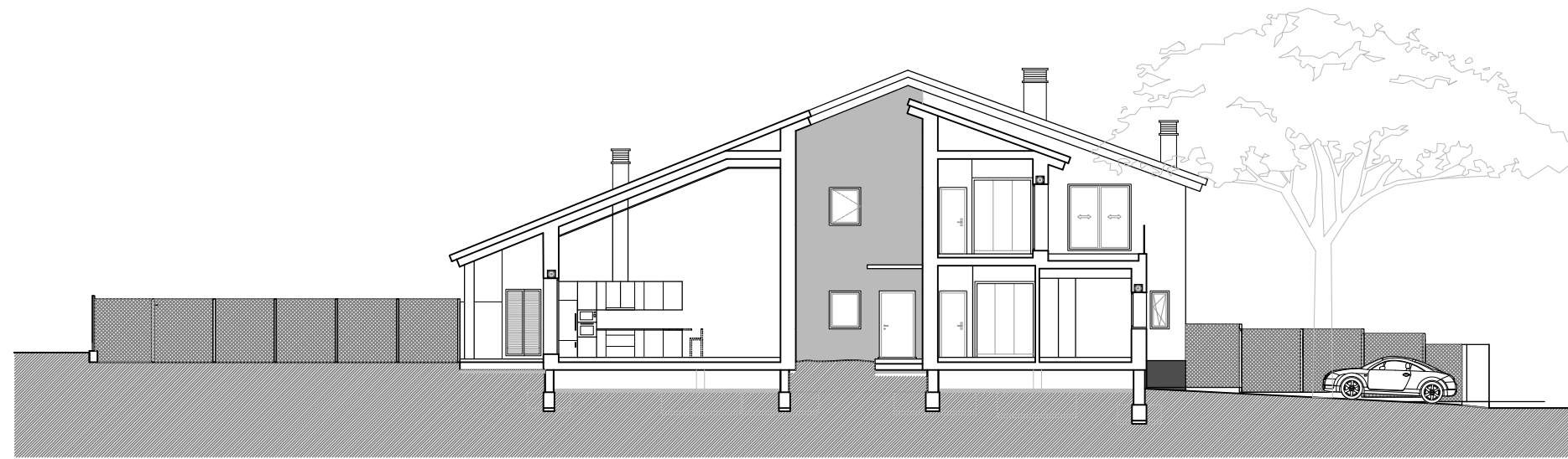
SECCIÓN ESQUEMÁTICA
