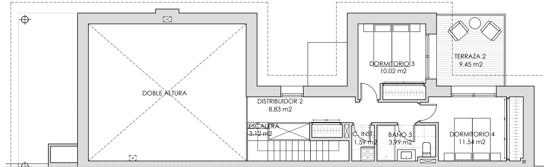
PLANTA PRIMERA
