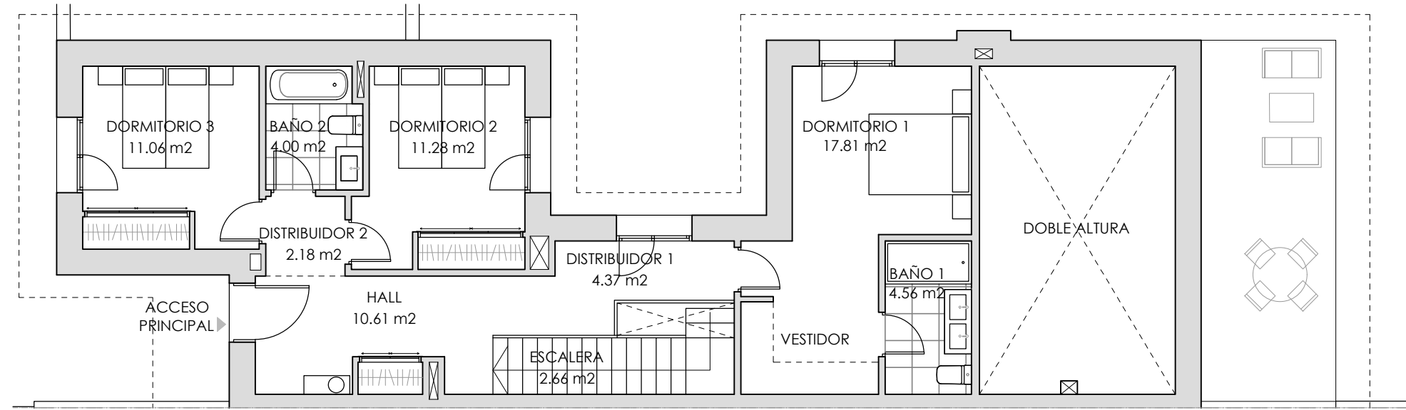
PLANTA PRIMERA
