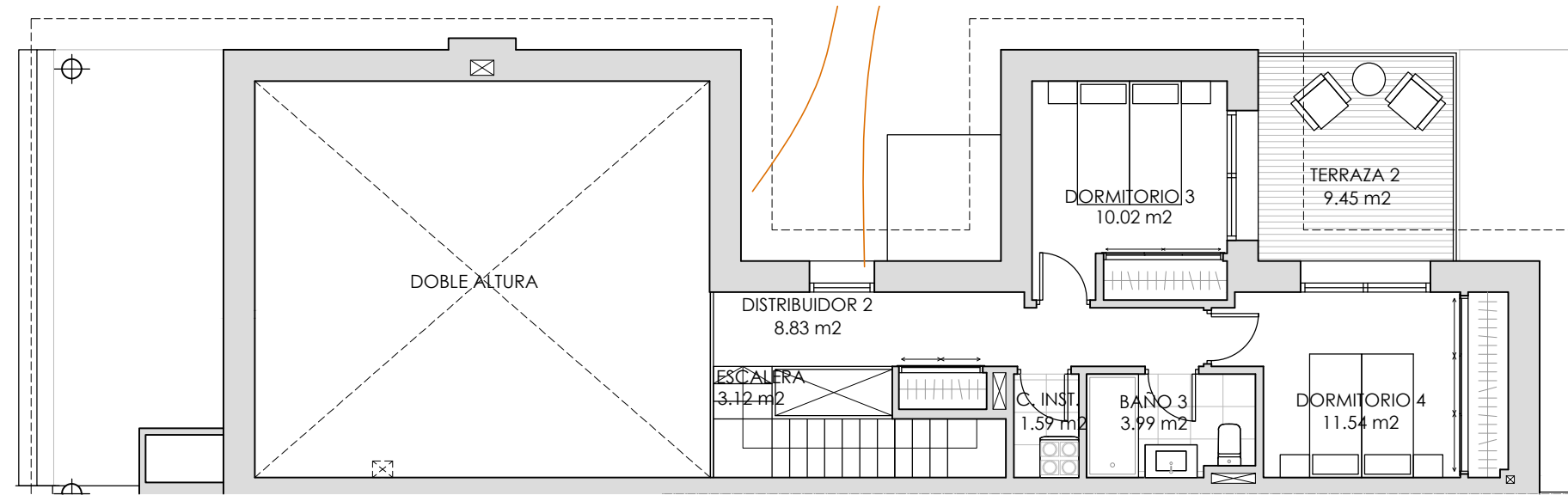
PLANTA PRIMERA
