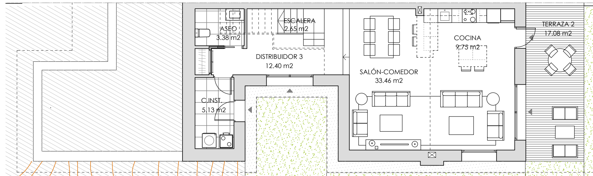
PLANTA BAJA
