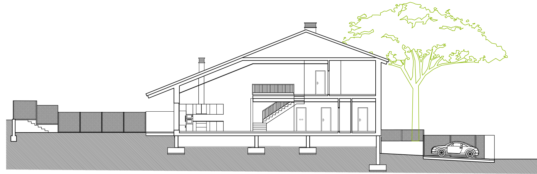
SECCIÓN ESQUEMÁTICA
