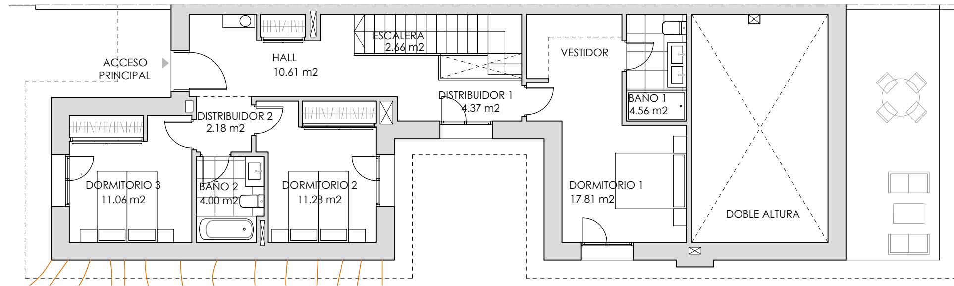
PLANTA PRIMERA
