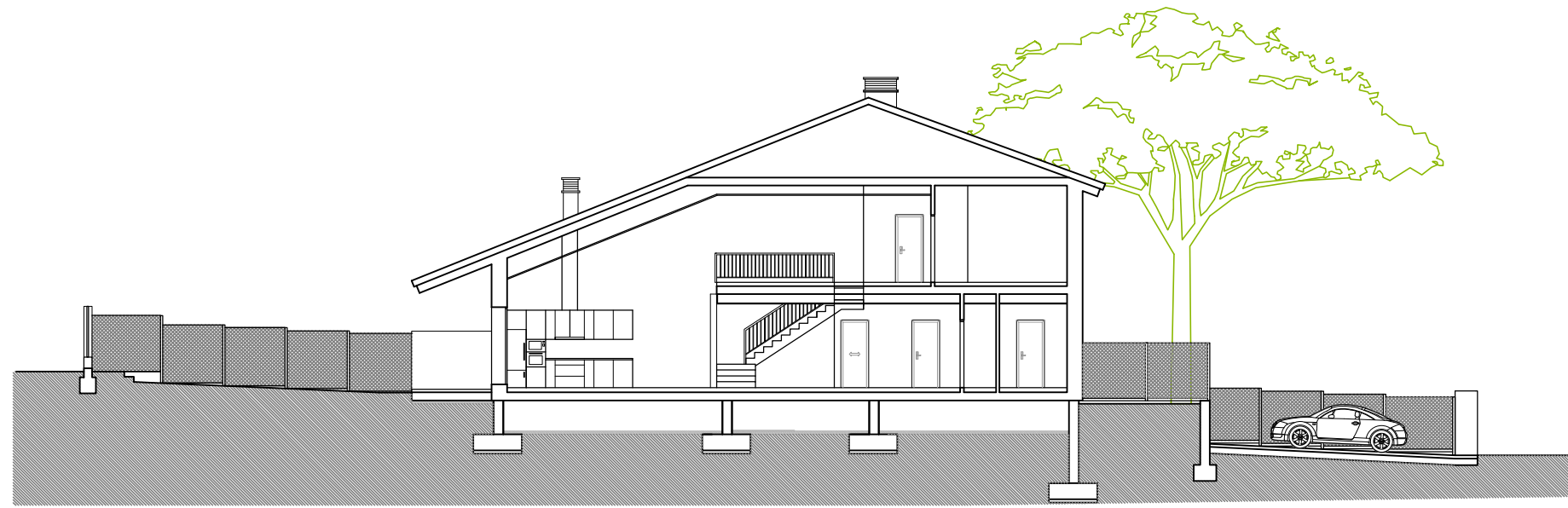
SECCIÓN ESQUEMÁTICA
