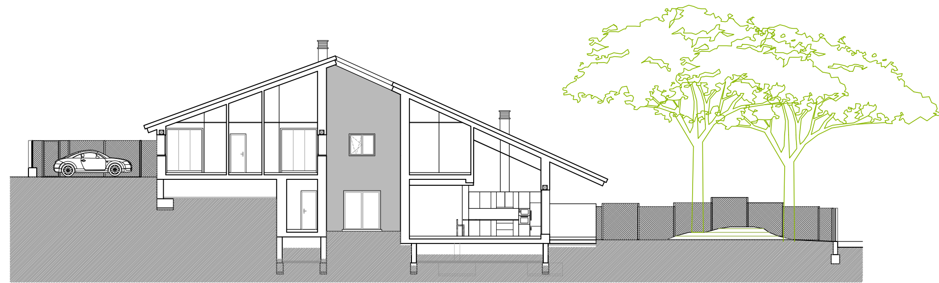
SECCIÓN ESQUEMÁTICA
