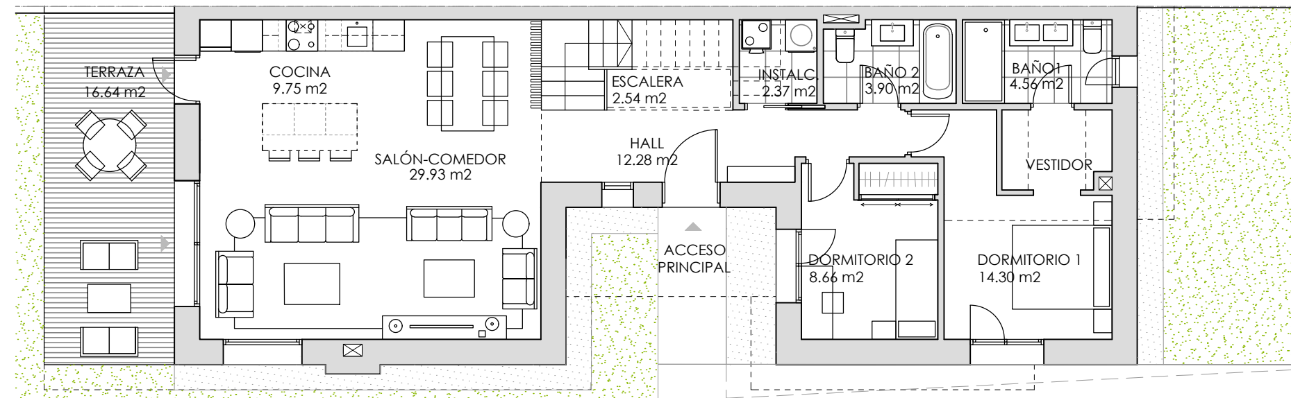
PLANTA BAJA
