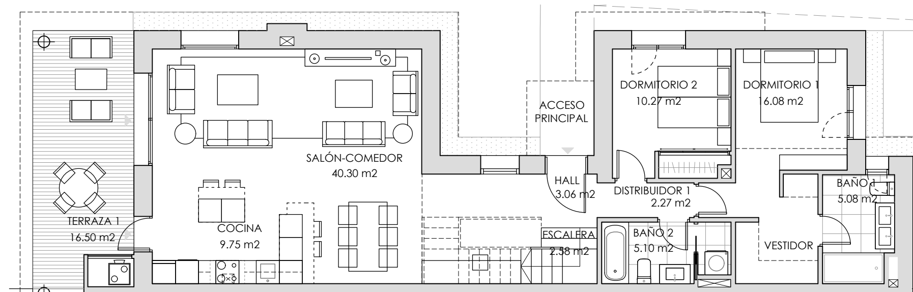
PLANTA BAJA
