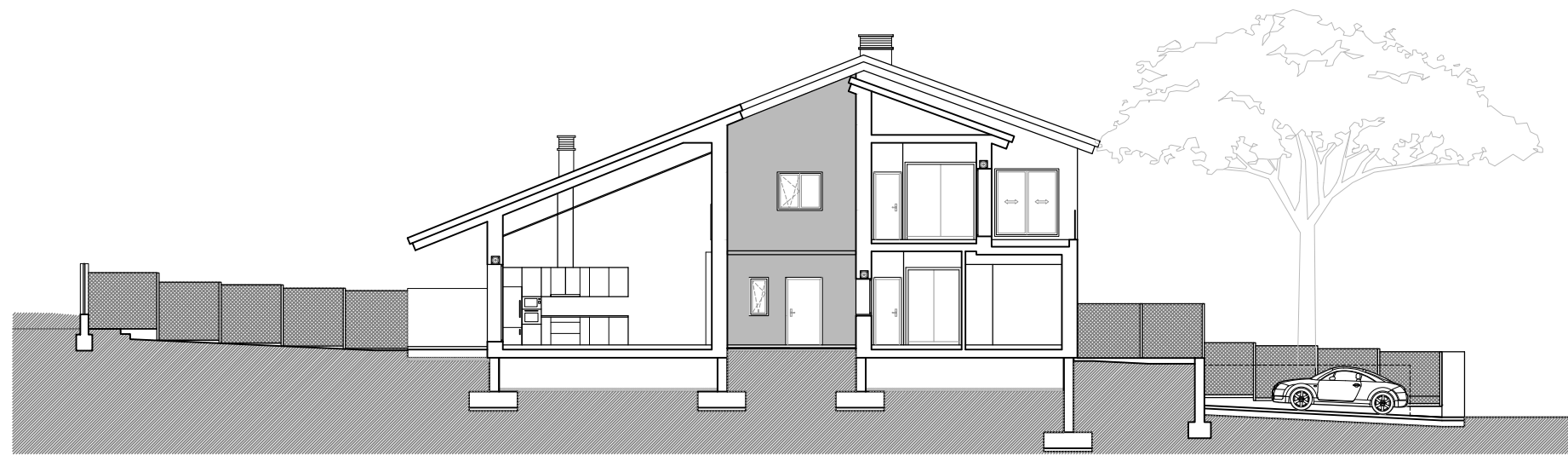
SECCIÓN ESQUEMÁTICA
