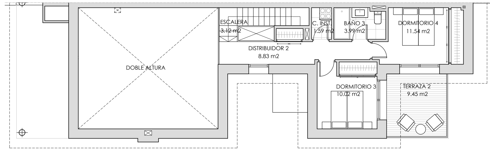
PLANTA PRIMERA
